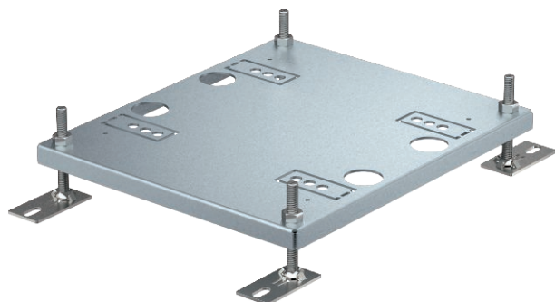
Регулируемая опора для увеличения высоты монтажа лючка UDHOME9.
