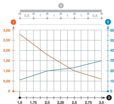
Диаграмма нагрузки на кабельный лоток лестничного типа SLZ
