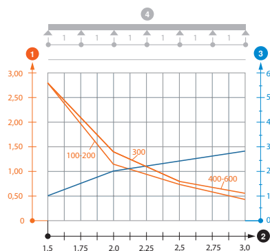
Диаграмма нагрузки на кабельный лоток лестничного типа SL62
