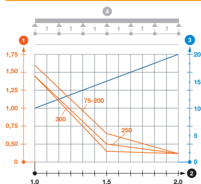
Диаграмма нагрузки на кабельный лоток лестничного типа SL42
