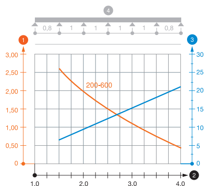
Диаграмма нагрузки SLG 60 NS
