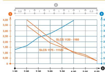
Диаграмма нагрузки на кабельный лоток лестничного типа SLCS 110
