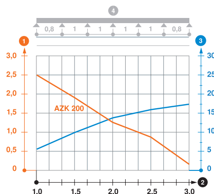
Диаграмма нагрузки на мини-канал AZ
