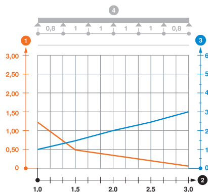
Диаграмма нагрузки на кабельный лоток RKS 35
