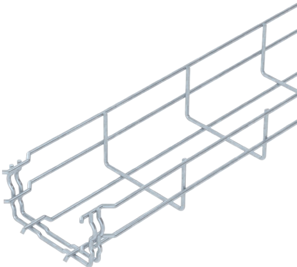
Проволочный лоток с соединителем соответствующей формы со сторонами высотой 55 мм.
