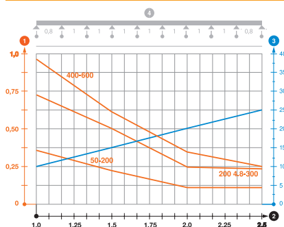
Диаграмма нагрузки на проволочный лоток GRM 55 VA
